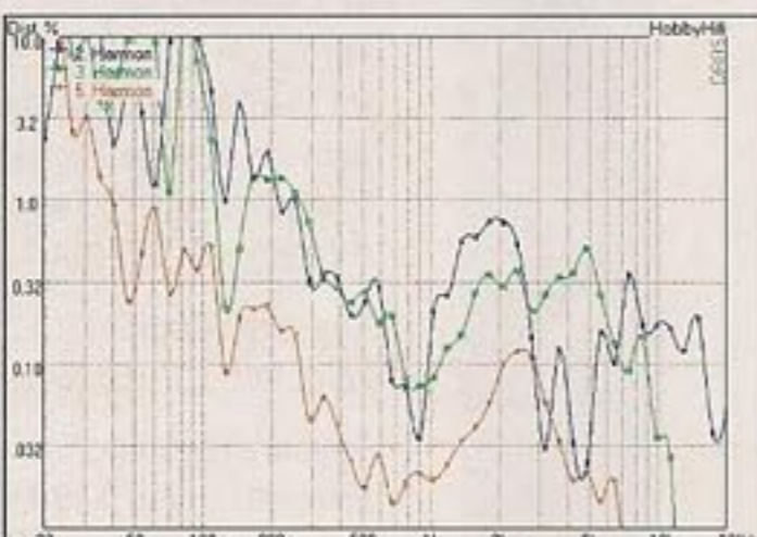
Klirrfaktor-Frequenzgänge K2, K3 u. K5 bei 90 dB mittlerem Schalldruckpegel mit Korrekturschaltung
