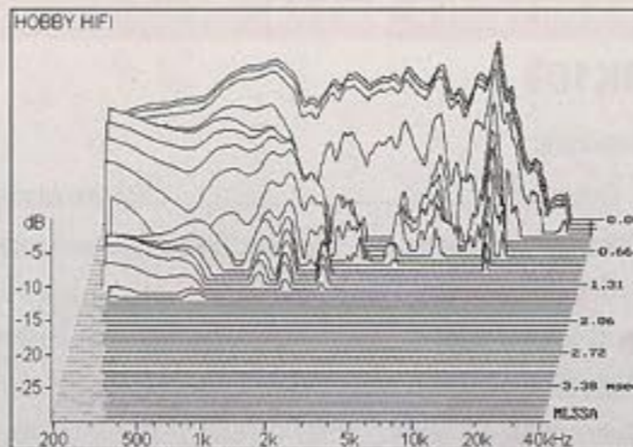
Wasserfallspektrum 0° ohne Korrekturschaltung
