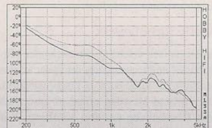
Phasenfrequenzgang ohne (...) und mit (...) Korrekturschaltung
