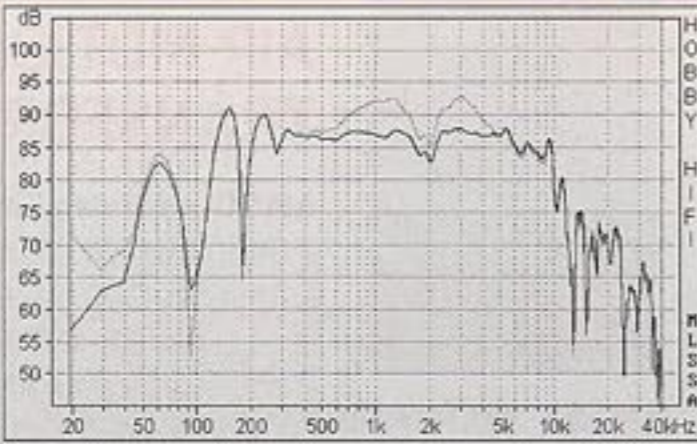
Schalldruck-Frequenzgang ohne (...) und mit (...) Korrekturschaltung unter 30°
