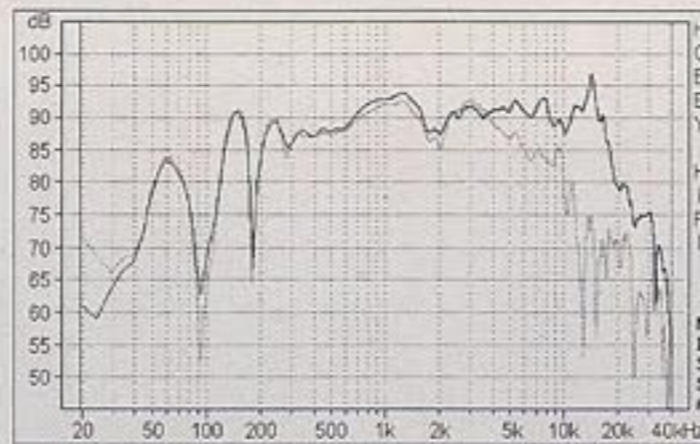
Schalldruck-Frequenzgang axial (...) und unter 30 Grad (...) ohne Korrekturschaltung
