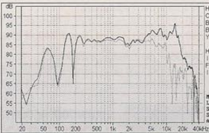
Schalldruck-Frequenzgang axial (...) und unter 30 Grad (...) mit Korrekturschaltung
