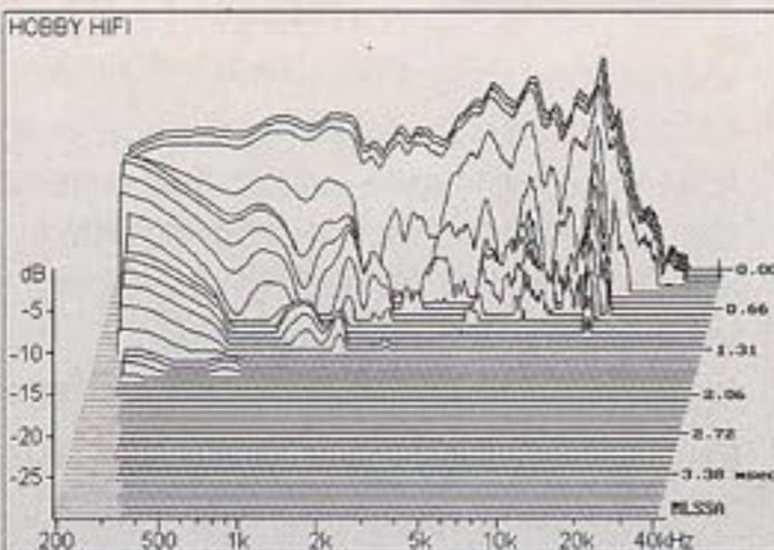
Wasserfallspektrum 0° mit Korrekturschaltung
