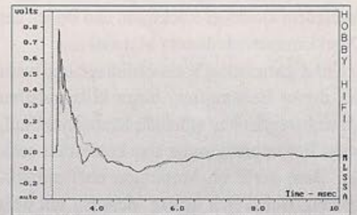
Sprungantwort 0° ohne (...) und mit (...) Korrekturschaltung
