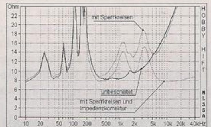
Impedanz-Frequenzgang unbeschaltet, mit Korrekturschaltung sowie mit Korrekturschaltung und Impedanzkorrektur
