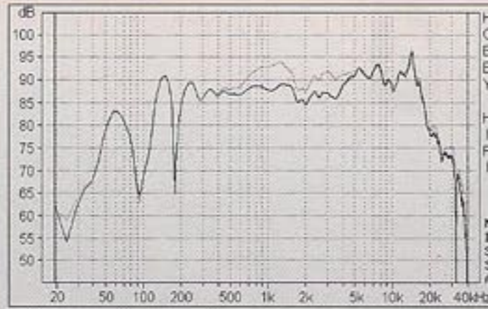
Schalldruck-Frequenzgang ohne (...) und mit (...) Korrekturschaltung axial
