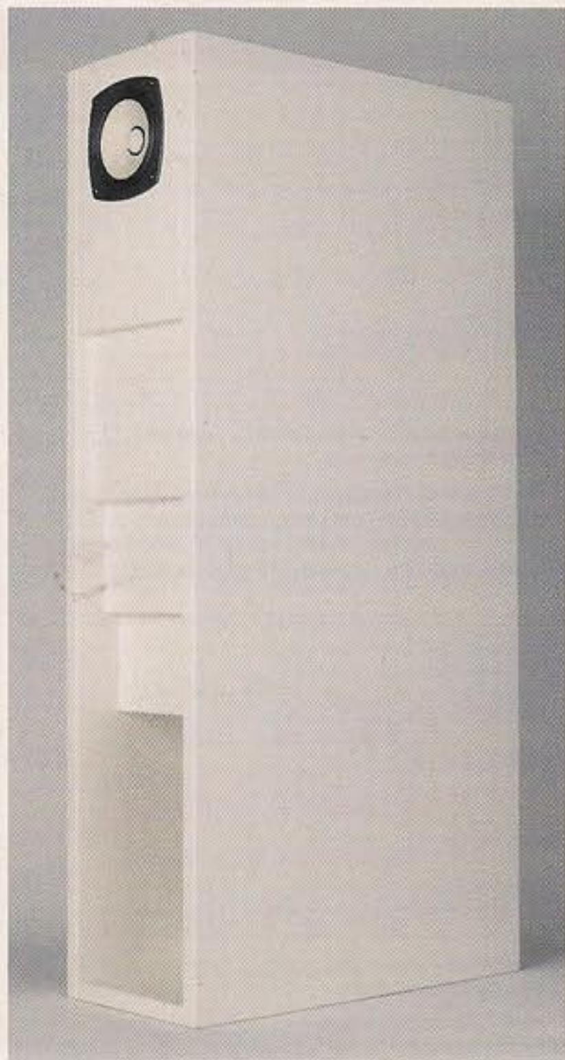
Das BK103 ist schlank, aber seine Tiefe nicht unerheblich: 40 Zentimeter tief baut das Horngehäuse, das einen 2,5 Meter langen Hornverlauf beherbergt.
