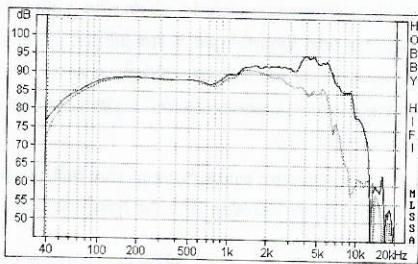
Exzellente Linearität, weitgehend resonanzfreier Roll-off.
